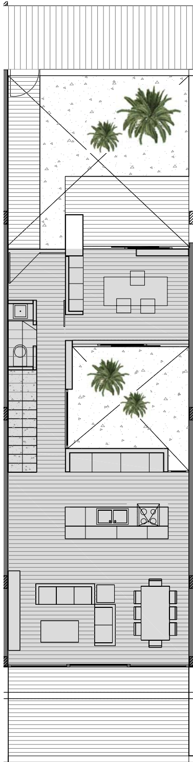
planta baja
