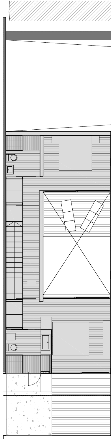
planta alta
